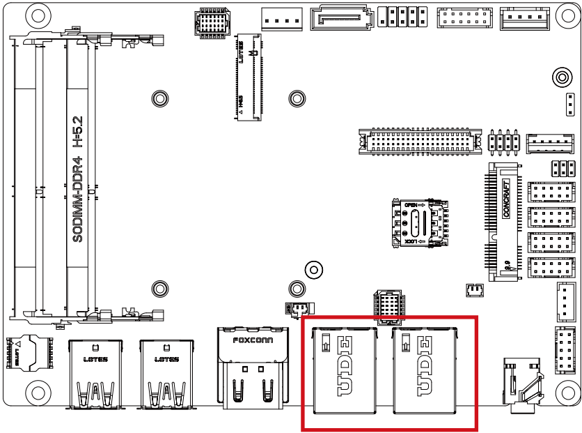
LAN Connector
