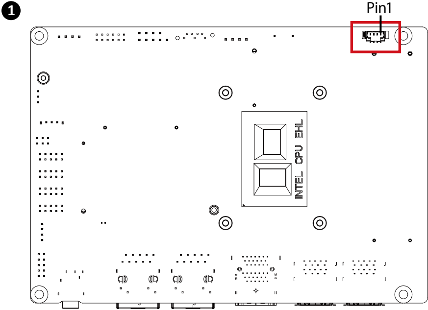
CPU/System FAN
