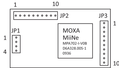
Bottom Panel of the MiiNePort E2 Module
