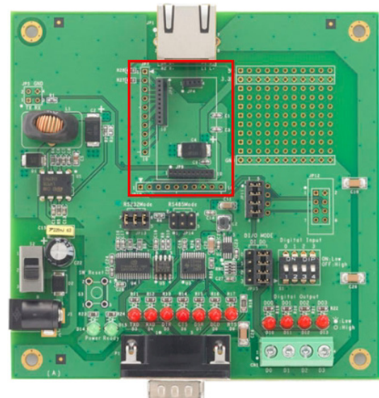
MiiNePort E2
